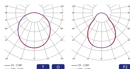
КРИВАЯ СИЛЫ СВЕТА
